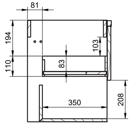
B-B ( 1 : 10 )
